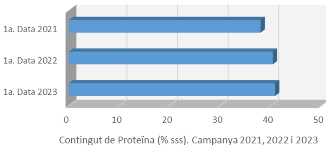
Figura 1. Contingut de proteïna del gra mitjà dels assaigs de les campanyes 2021, 2022 i 2023.
