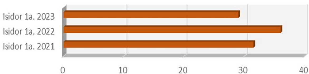
Durada de la floració de ISIDOR (dies). Campanya 2021, 2022 i 2023
