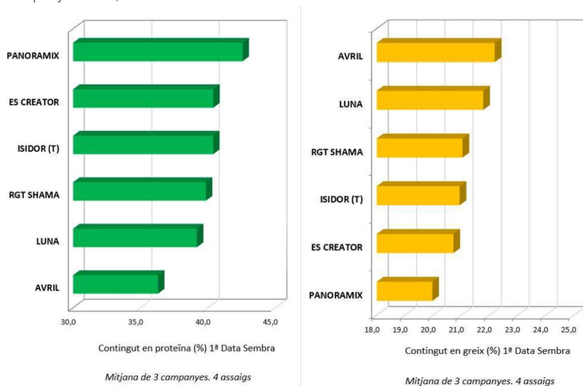
Figura 3. Contingut de proteïna i greix del gra. Valors mitjans per varietat. Cicles llargs, 1a data de sembra. Sucs (el Segrià). Campanyes 2021, 2022 i 2023.
