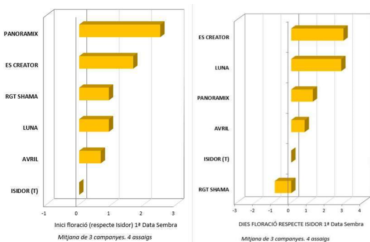
Figura 4. Inici de floració i durada de la floració (dies respecte la varietat ISIDOR). Assaigs de varietats en primera data de sembra, cicles llargs. Sucs (el Segrià). Campanyes 2021, 2022 i 2023.
